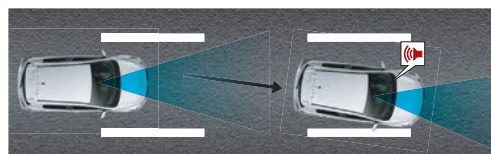
Avertizare + frânare automată puternică
